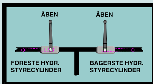
Omskifters under låseplade for hydraulisk styring
