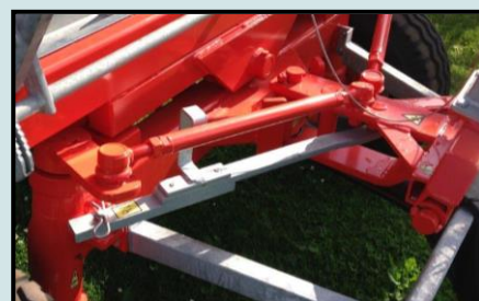
Manuel styring med låsepal monteret.
