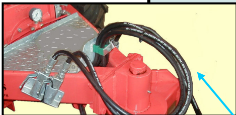
Slanger for hydraulisk bremse og hydraulisk styrecylinder (ekstraustyr).
