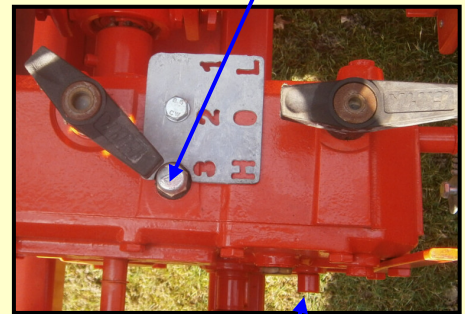
Prop for olieniveau.
